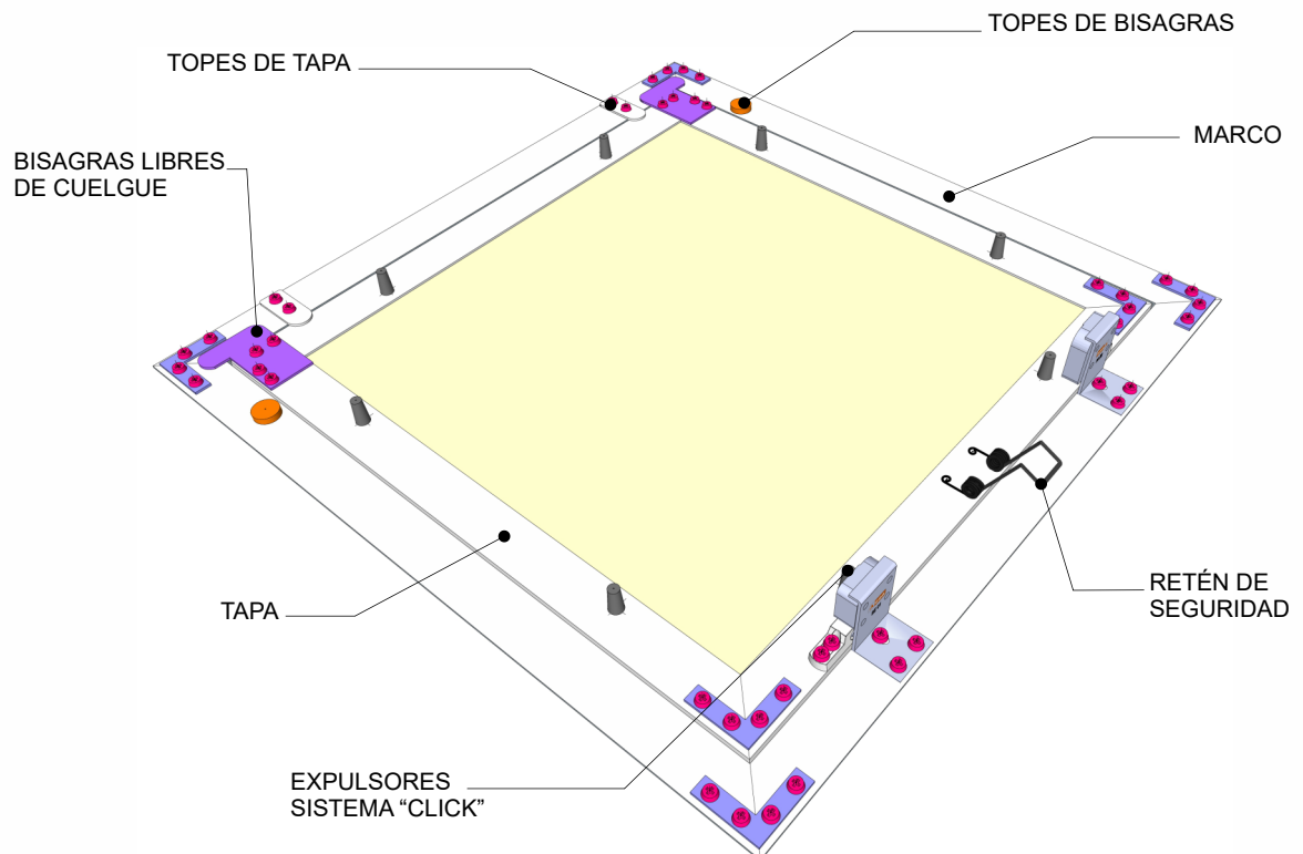
tapa cerrada
