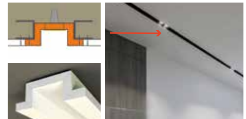
RIS 2 (Cielorraso)
